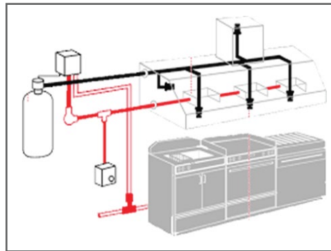
نظام إخماد حريق المطابخ KITCHEN FIRE SUPPRESSION SYSTEM
